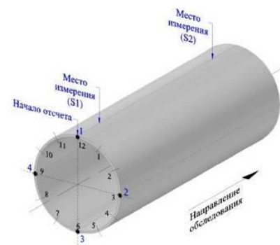
Рисунок 1 – Схема проведения измерения толщины стенки
